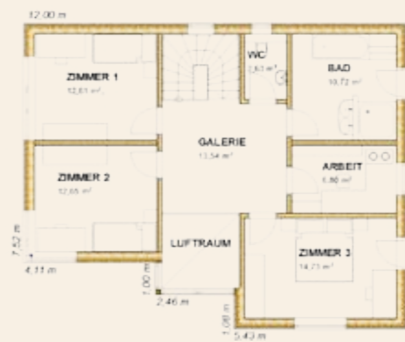
Dachgeschoss
