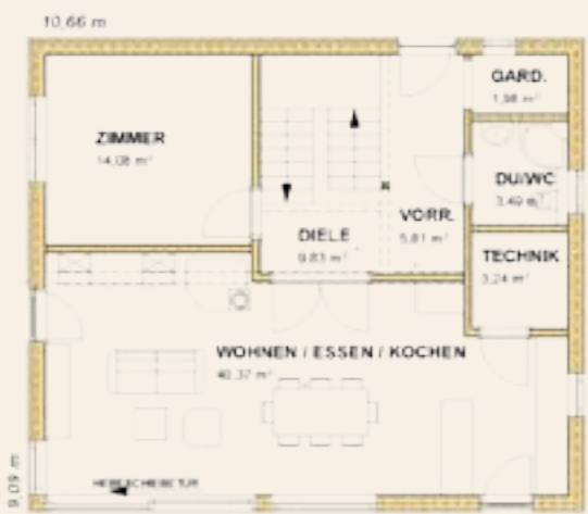
Erdgeschoß
